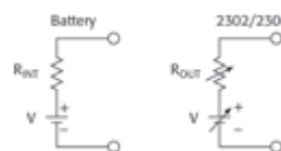
Упрощенная эквивалентная схема батареи и источника питания 2302/2306.
