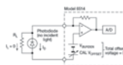
Применение модели 6514 для измерения темного тока фотодиода.
