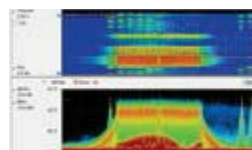
Спектр DPX
